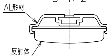
A - A' 断面図 S = 1 / 2
