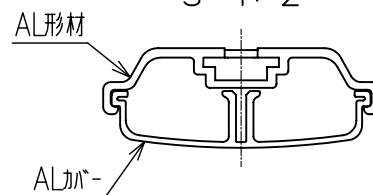
B - B' 断面図 S = 1 / 2
