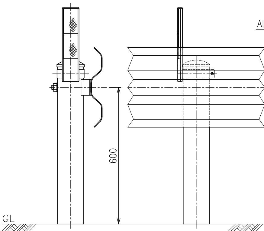
設置図 S = 1 / 10
