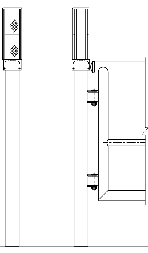
設置図 S=1/10
