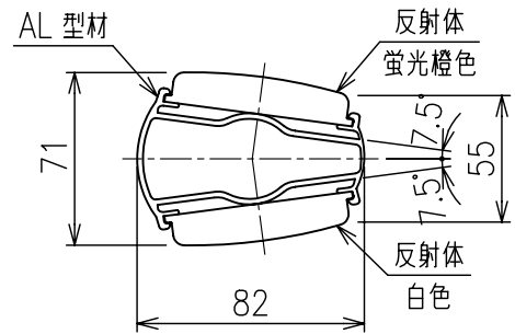
A-A' 断面図 S=1/3
