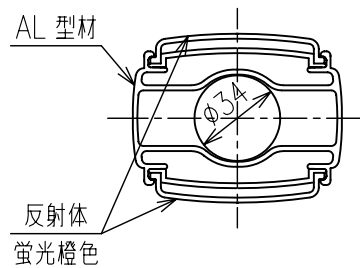
A - A' 断面図 S=1/3
