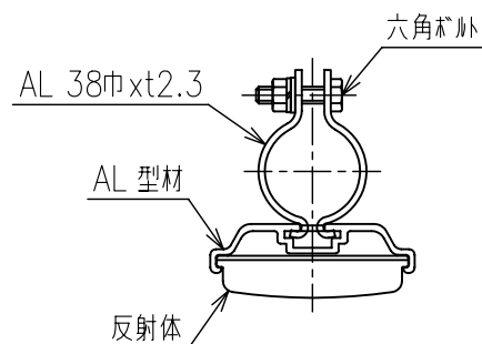
A - A' 断面図 S=1/3
