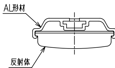
A - A' 断面図 S=1:2
