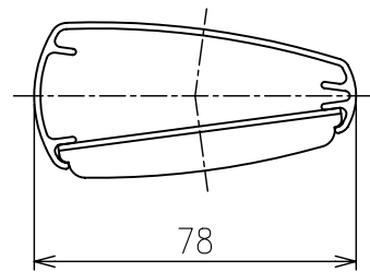
A - A' 断面図 S=1/2
