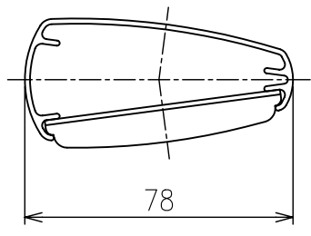
A - A' 断面図 S=1/2
