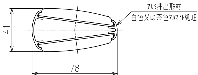
A - A' 詳細図 S=1/2
