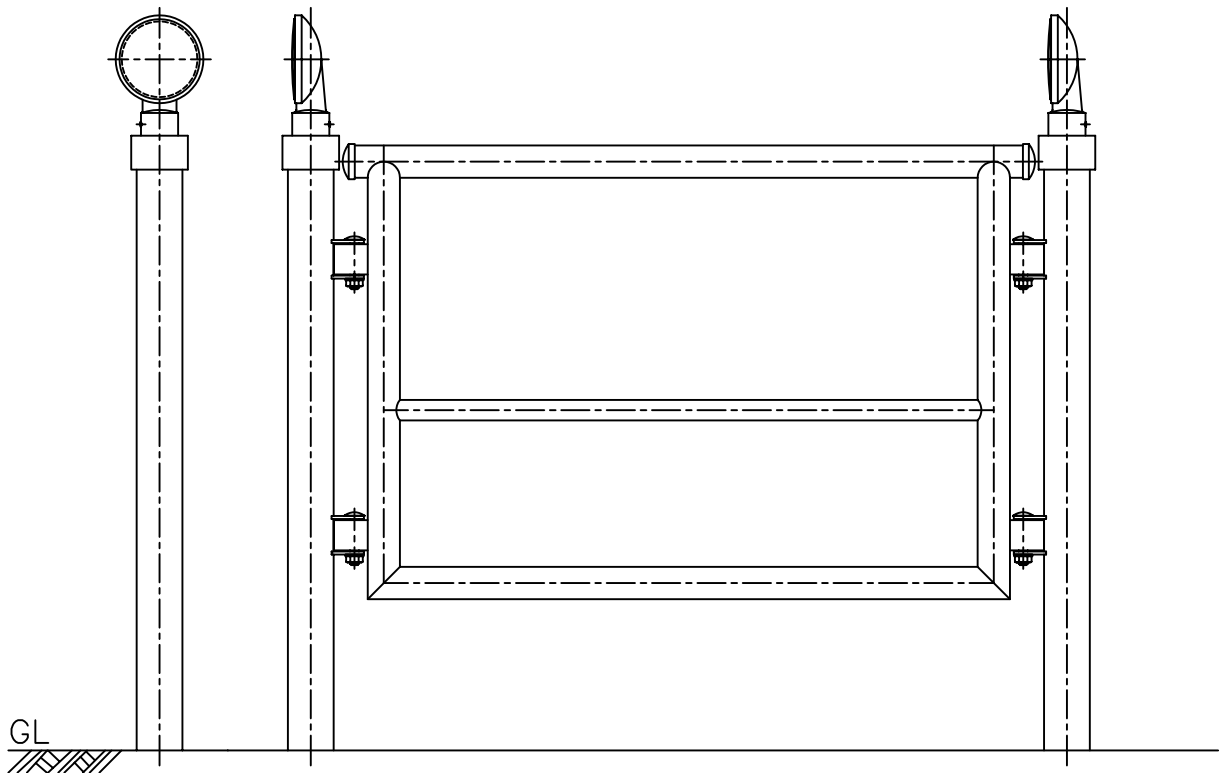
設置図 S=1/10
