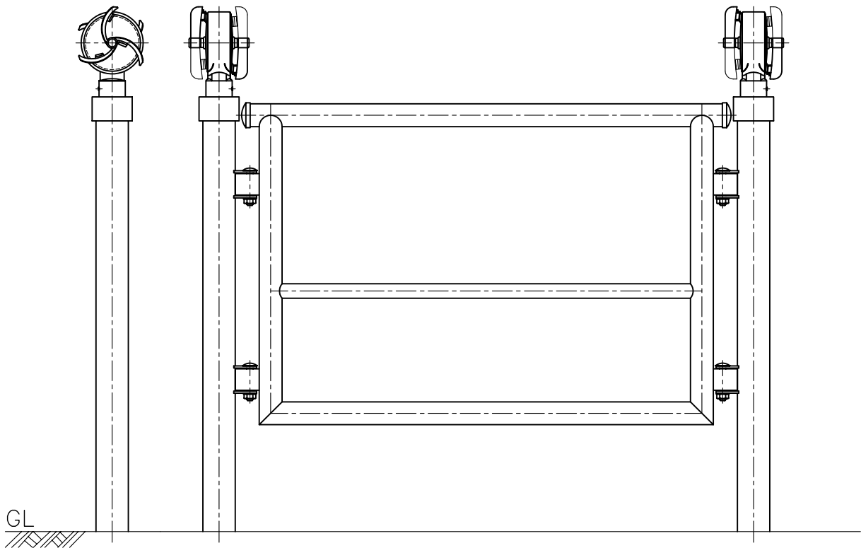
設置図 S=1/10
