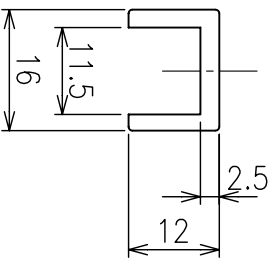
ヒート断面図 S=1/1
