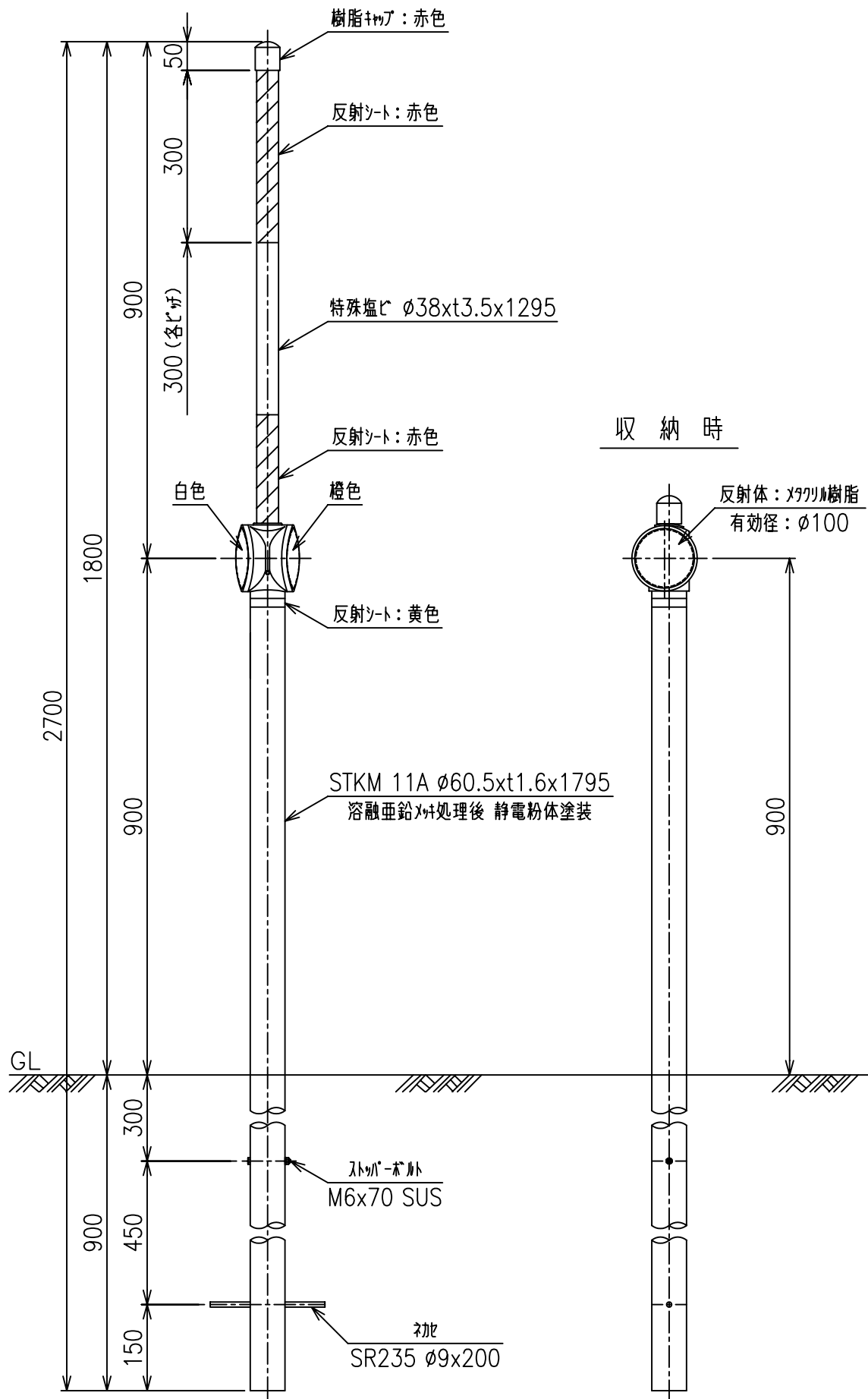
DWM-A-SP-100 (土中式 ひねり式) Scale 1/10 株式会社 カシマ
