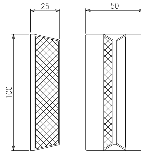
詳細図 S=1:2
