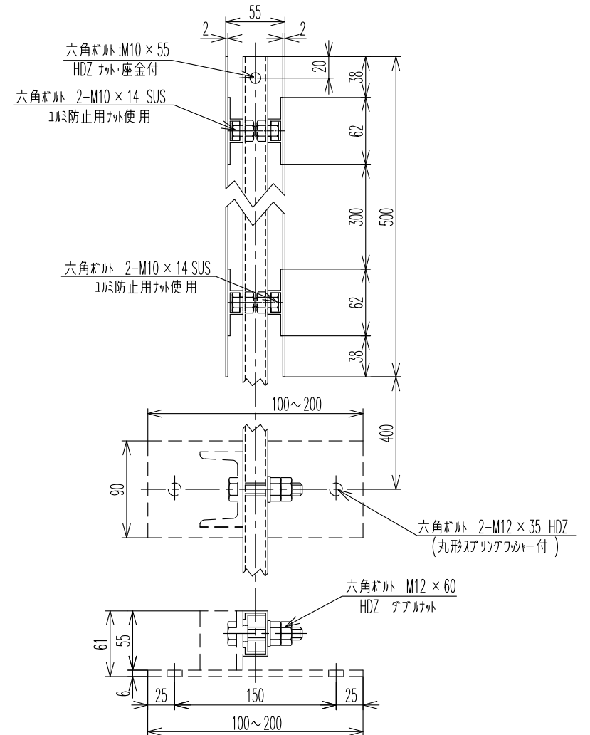
詳細図 S=1:5
