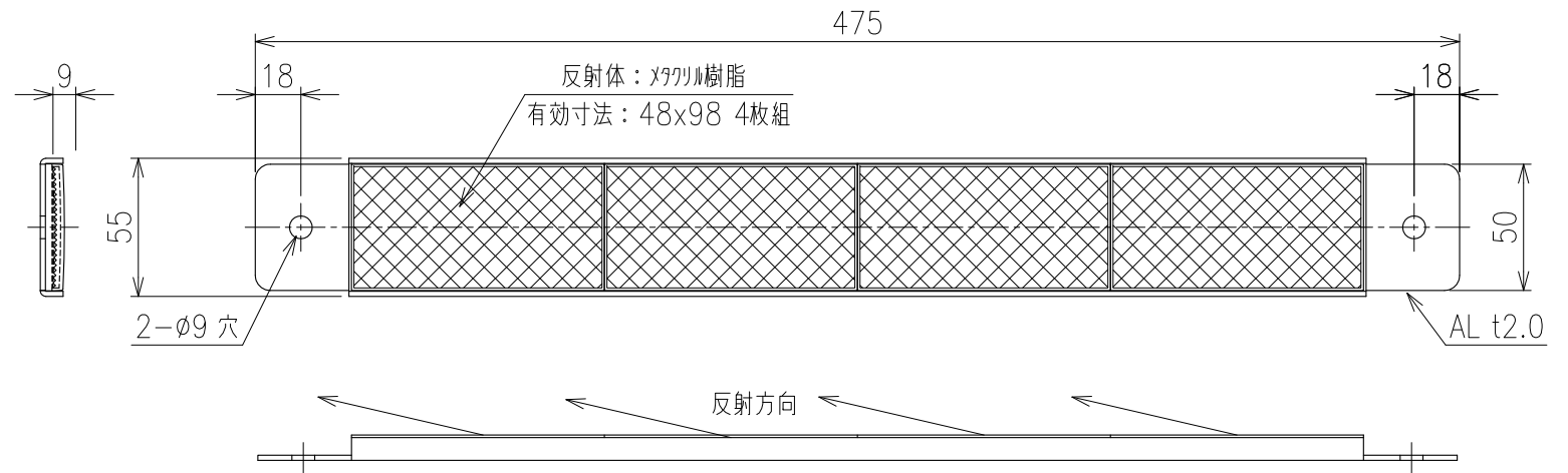
詳細図 S=1/3
