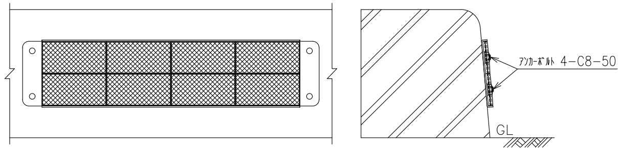
設置図 S=1:6
