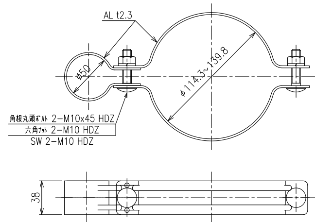
バンド詳細図 S=1:4
