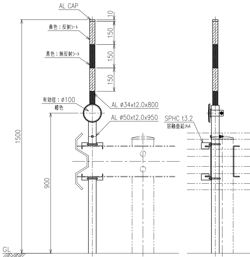
引っ掛け金具 S=1:7
