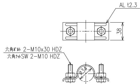
取付金具 S=1:4
