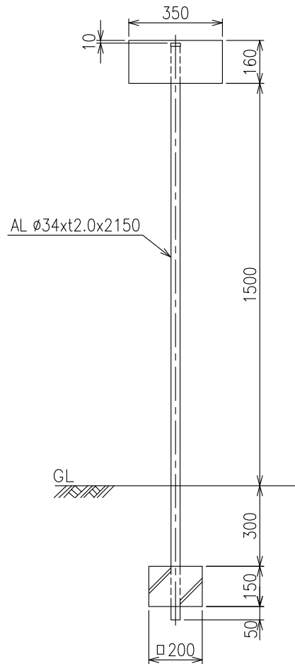
設置図 S=1:20
