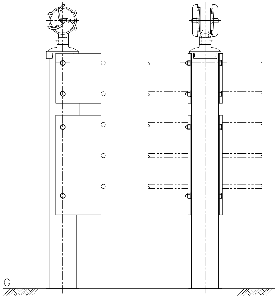
設置図 S=1:10
