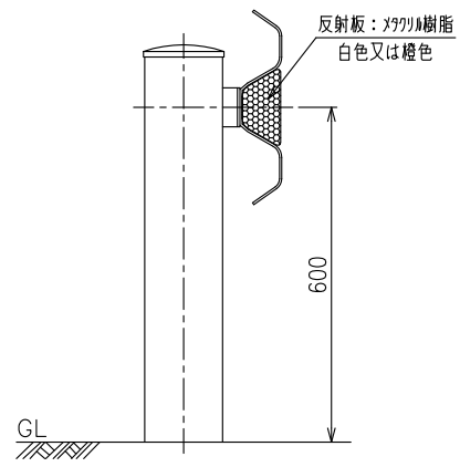
設置図 S=1:15
