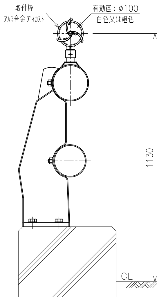
取付金具 詳細図
