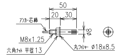
C8-50アンカー
