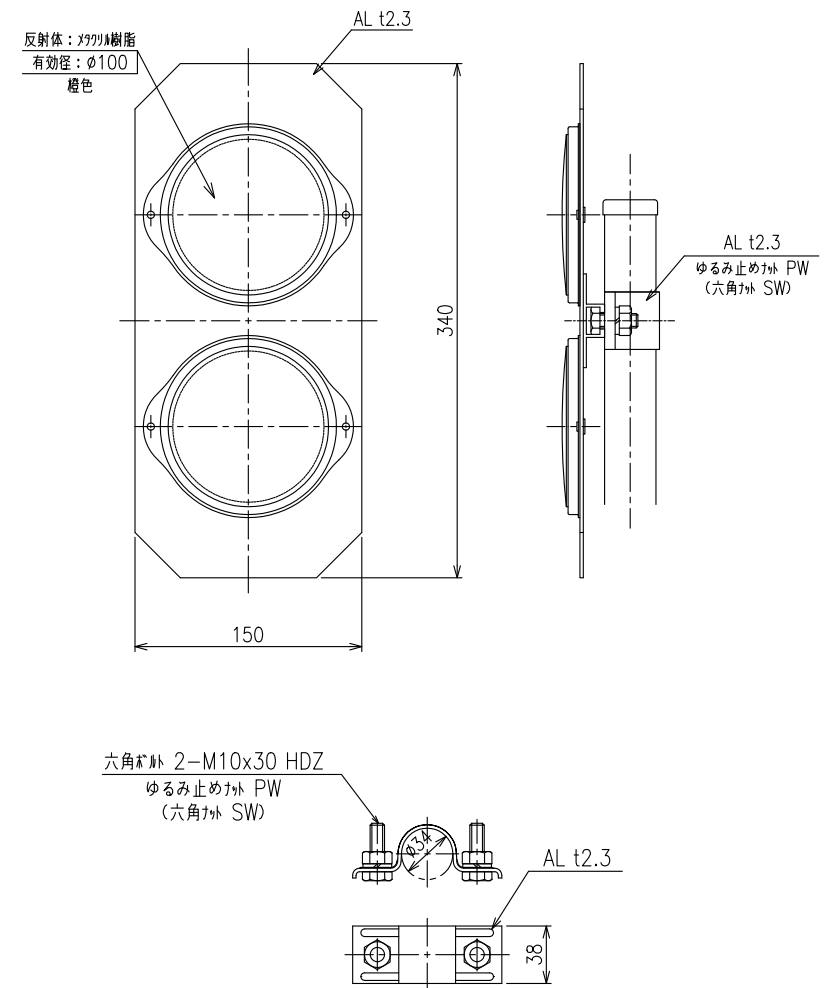
頭部詳細図 S=1:5
