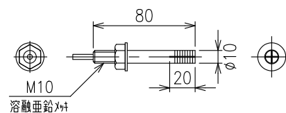
アンカー詳細図 S=1:4
