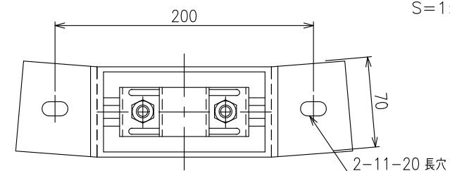
上下部取付金具 S=1:3
