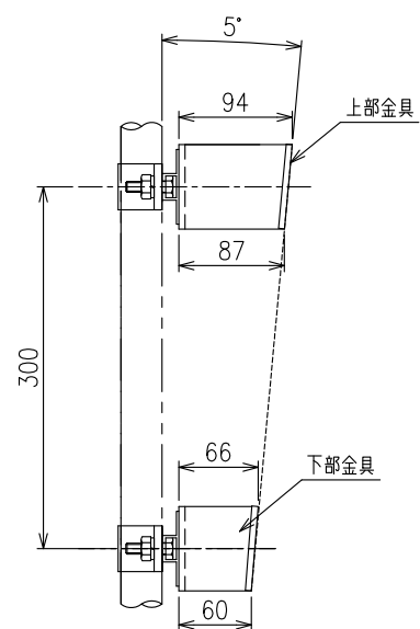
拡大図 S=1:5
