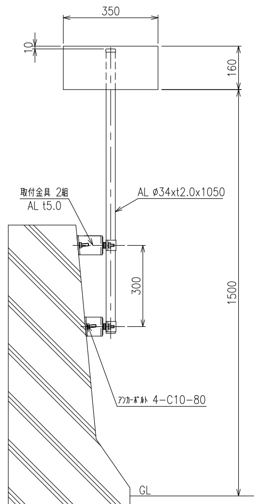
設置図 S=1:10
