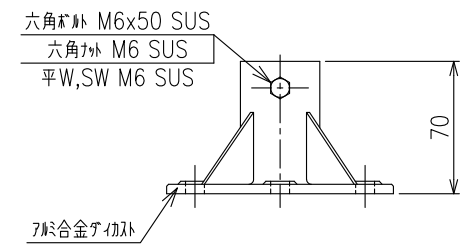
アジャスター詳細図
