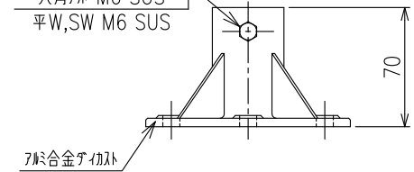
アジャスター詳細図
