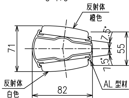
A-A' 断面図
