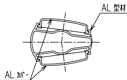
B-B' 断面図
