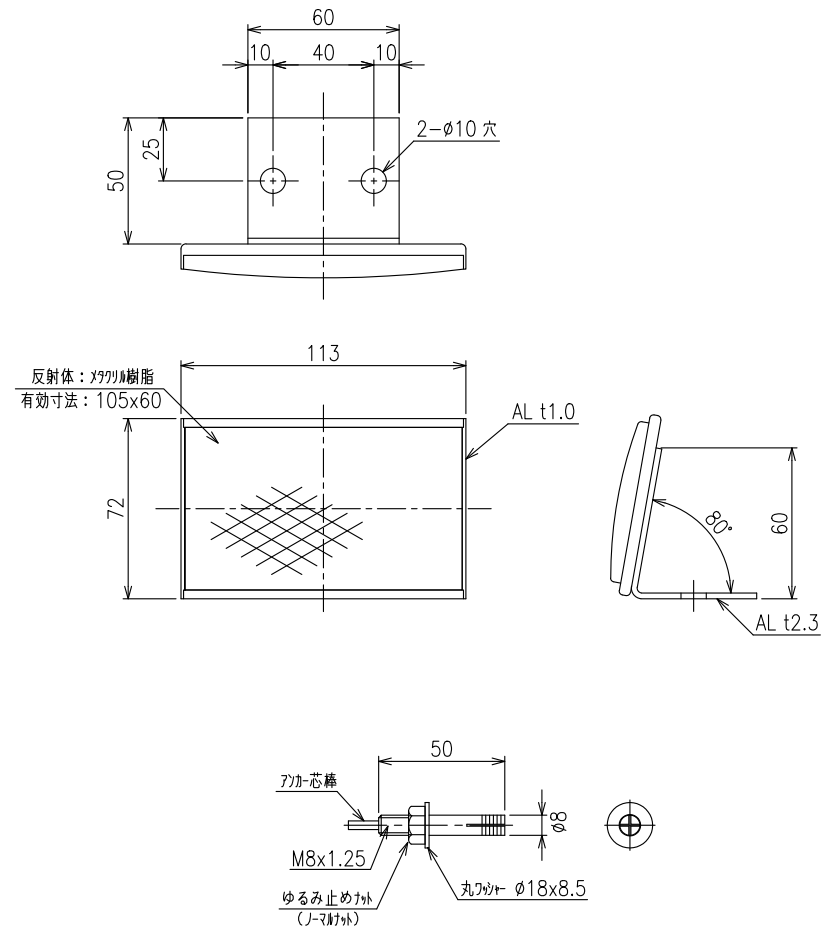
詳細図
