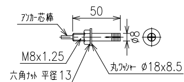
アジャ-詳細図 S=1:4
