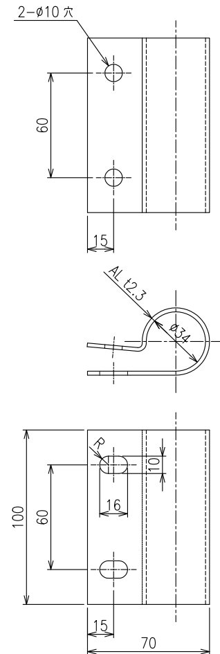
金具詳細図 S=1:3
