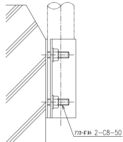
アジャ-詳細図 S=1:4
