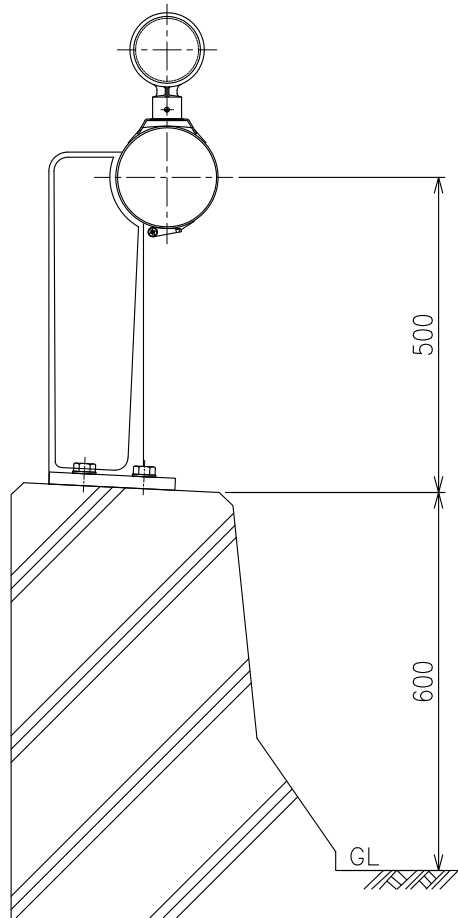
設置図 S=1:12
