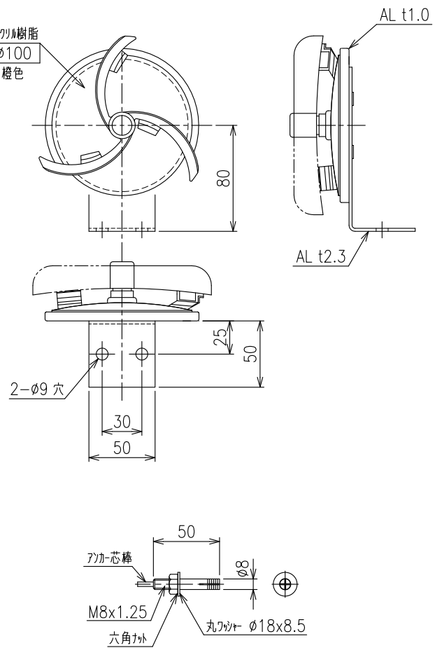
詳細図 S=1:4
