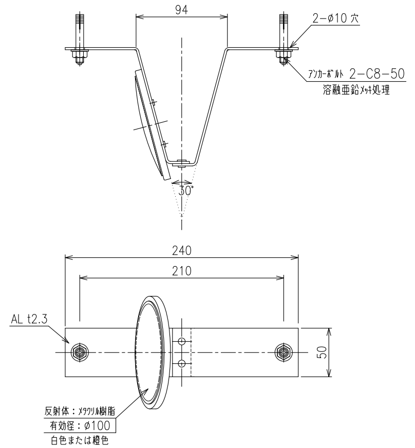
詳細図 S=1:4
