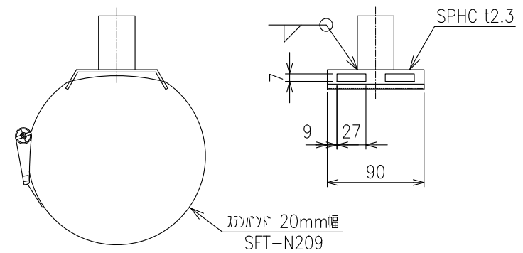
金具詳細図 S=1:5
