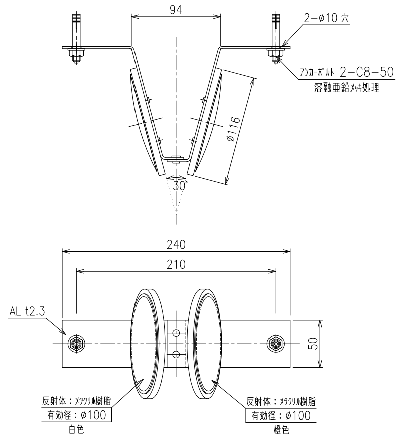
詳細図 S=1:4
