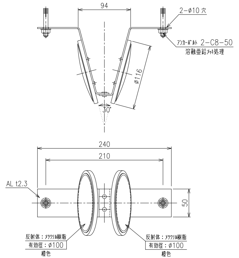
詳細図 S=1:4
