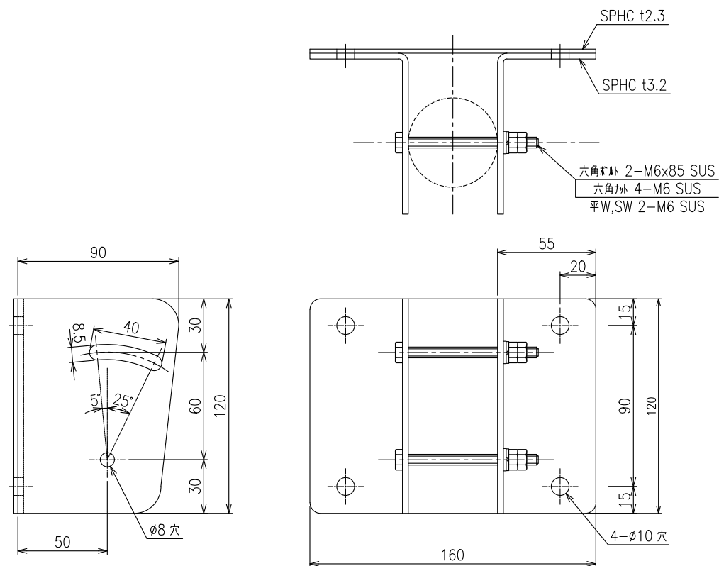
詳細図 S=1:3
