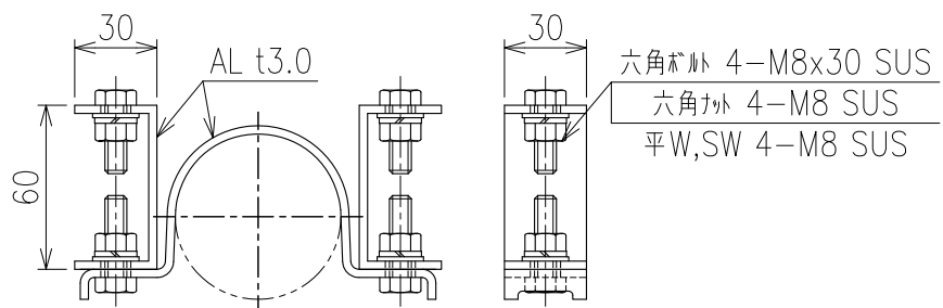
両面金具詳細図
