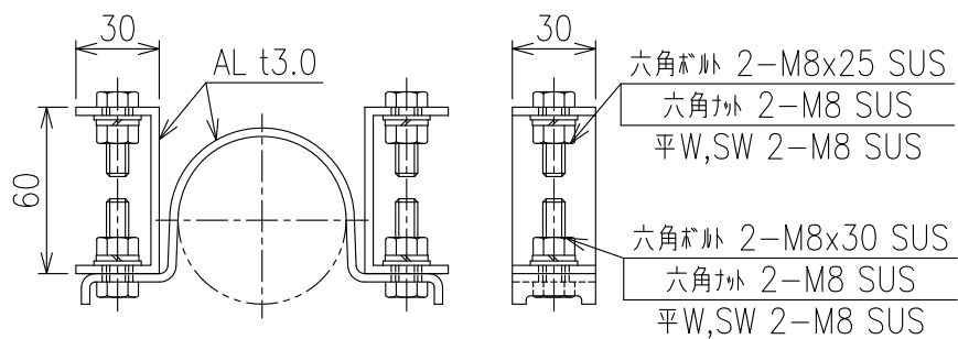
両面金具詳細図
