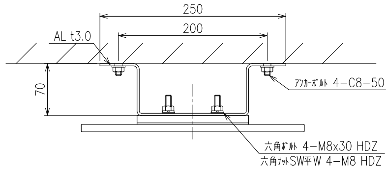
詳細図 S=1:5
