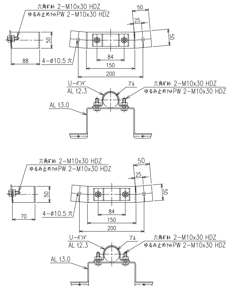
取付金具詳細図 S=1:7
