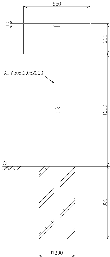
設置図 S=1:15
