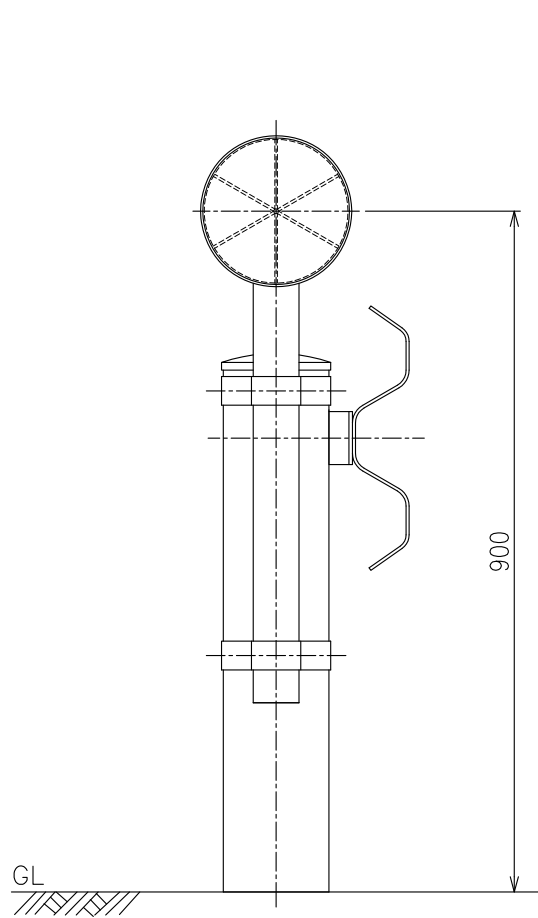
設置図 S=1:10
