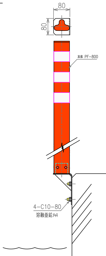
設置図 S=1:9
