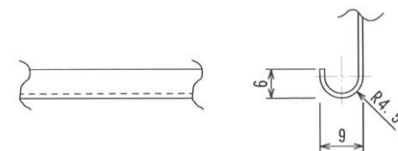
カーリング部詳細図 S=1:1
