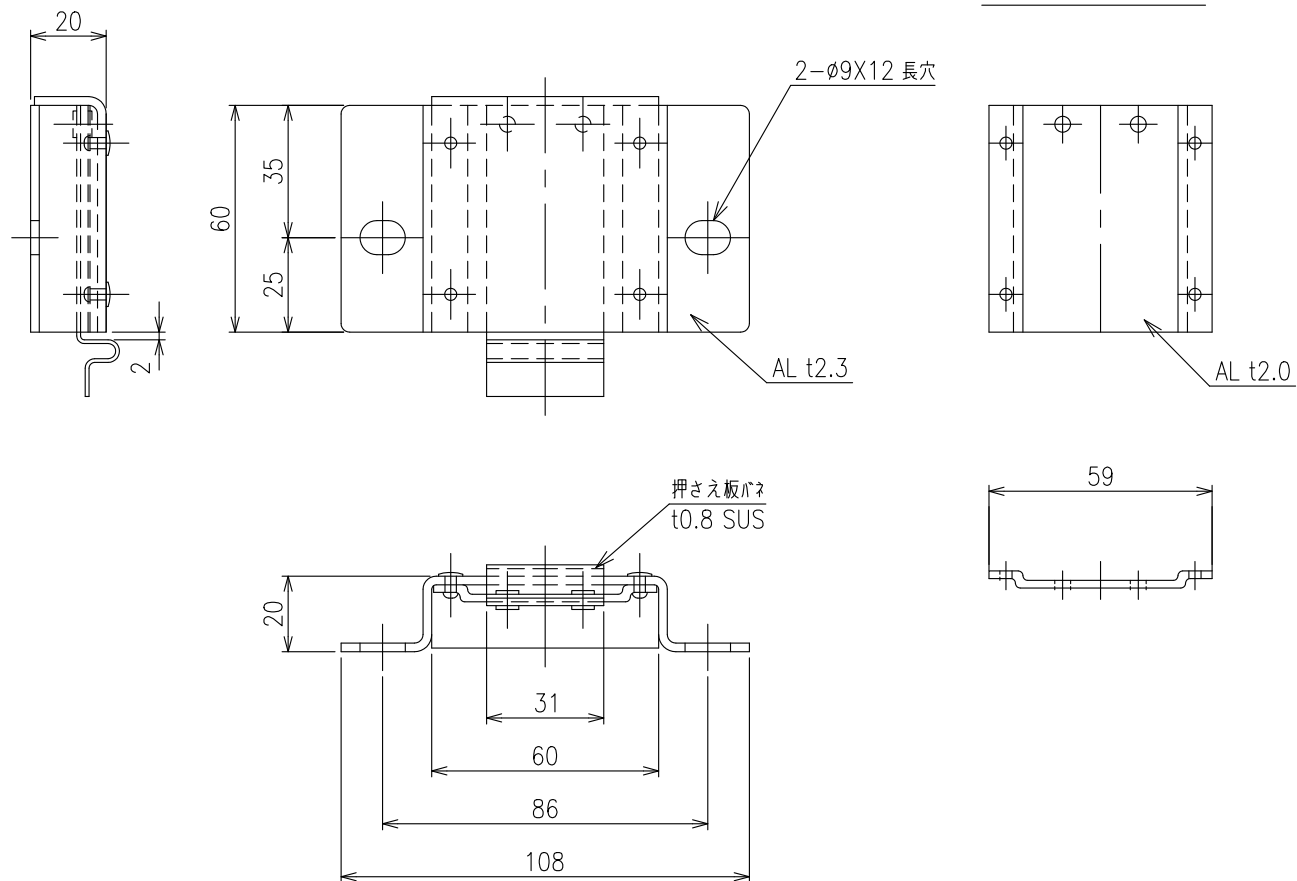
バネ取付板 詳細図
