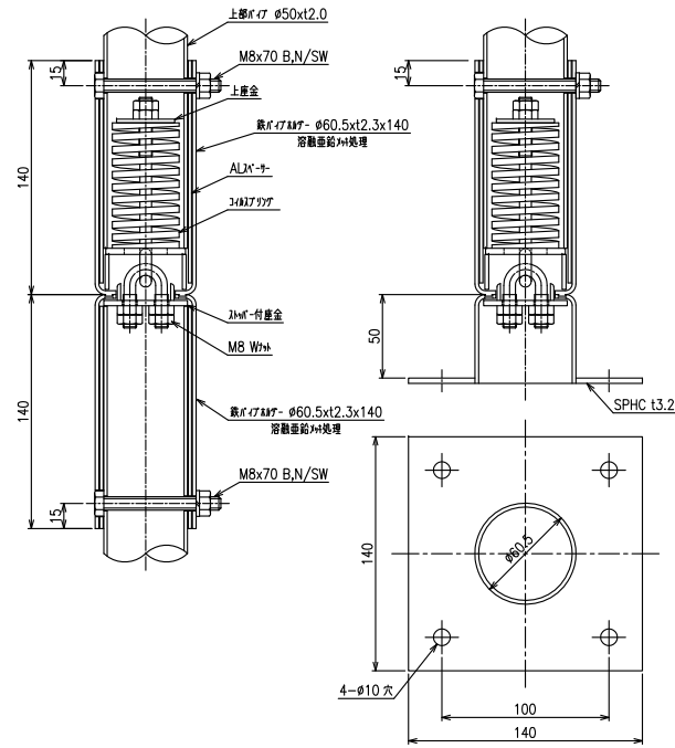
RV-50B φ50支柱ベース用
