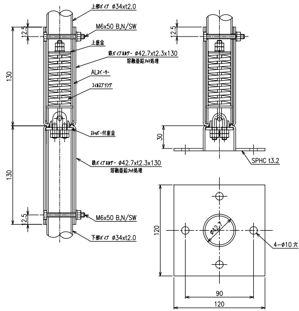
RV-34B φ34支柱ベース用
