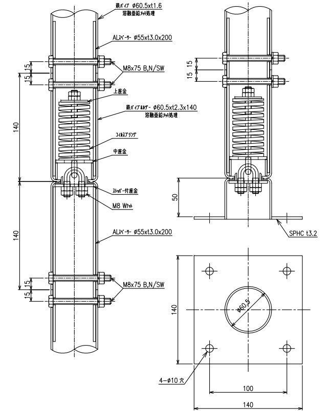
RV-60B φ60.5支柱ベース用
