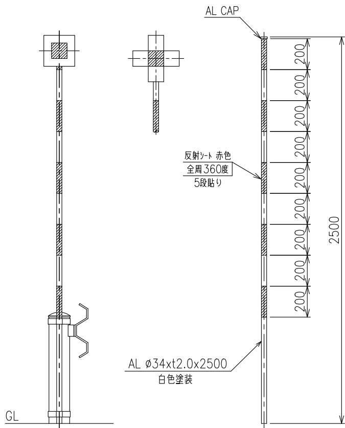
設置図
