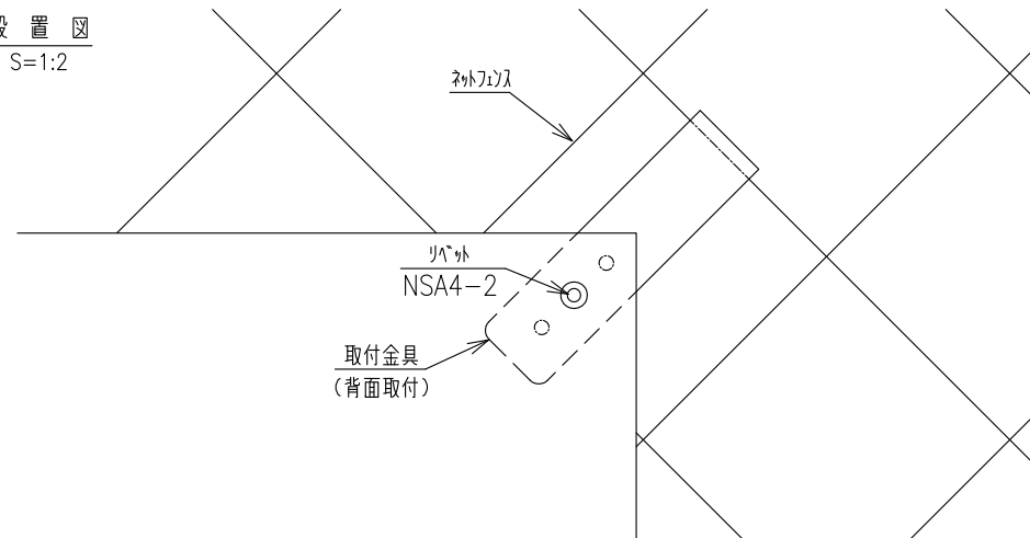
穴位置図
